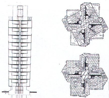
A LA IZQUIERDA, SECCIÓN Y PLANTAS DE LA TORRE DE SAINT MARK, DE WRIGHT. A LA DERECHA, ROTATIVAS DEL PERIODICO TURUN SANOMAT EN TURKU, DE AALTO. ABAJO, A LA IZQUIERDA, OFICINAS DE LA FABRICA JOHNSON, DE WRIGHT. ABAJO, A LA DERECHA, NAVE DE MAILLART.
