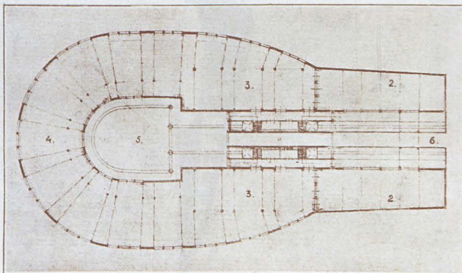
FÁBRICA DE ÓPTICA.
