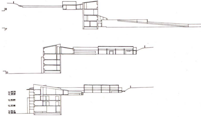
Secciones. Sections.
