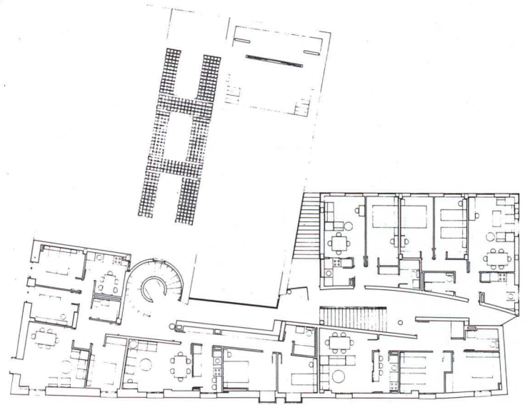
Planta viviendas. Plan of the housing.
