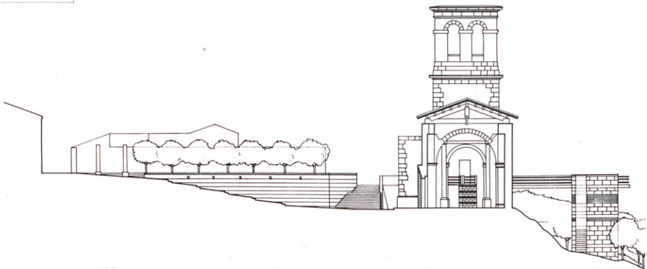
SECCIÓN A-A
