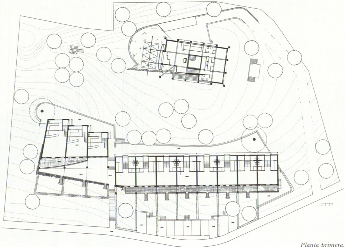
Planta primera.
