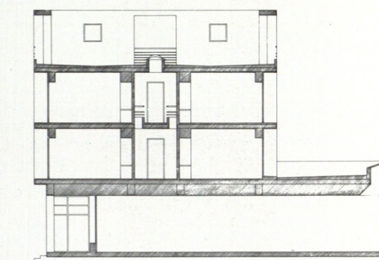
SECCION TRANSVERSAL
