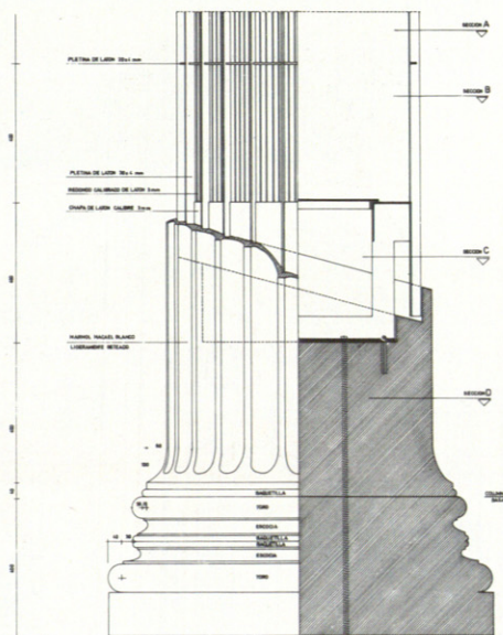
PAJARERA EN OSUNA DETALLE DE CONSTRUCCION E/15
