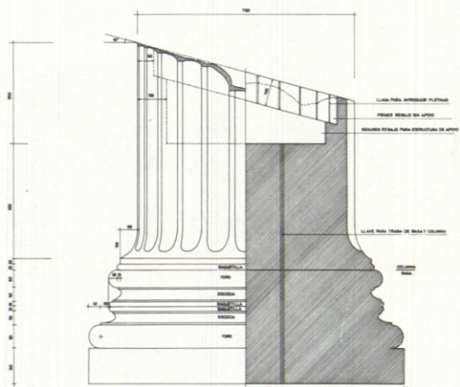
PAJARERA EN OSUNA DETALLE DE LA BASA Y COLUMNA E/15 escala 8x=1
