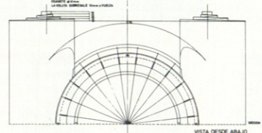
PAJARERA EN OSUNA DETALLE DE CONSTRUCCION DE CAPITEL E/15
