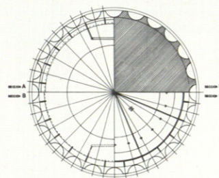
PAJARERA EN OSUNA DETALLE DE CONSTRUCCION DE CAPITEL E/15
