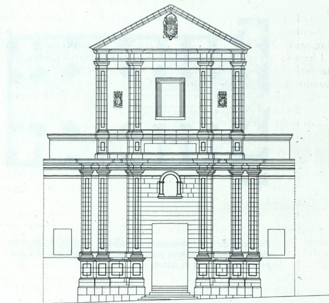
Parte construida de la fachada del siglo XVI.
