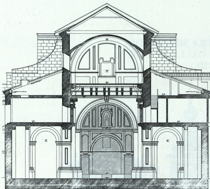
Sección longitudinal y planta en estado actual, con el hipotético trazado de la Iglesia completa.
