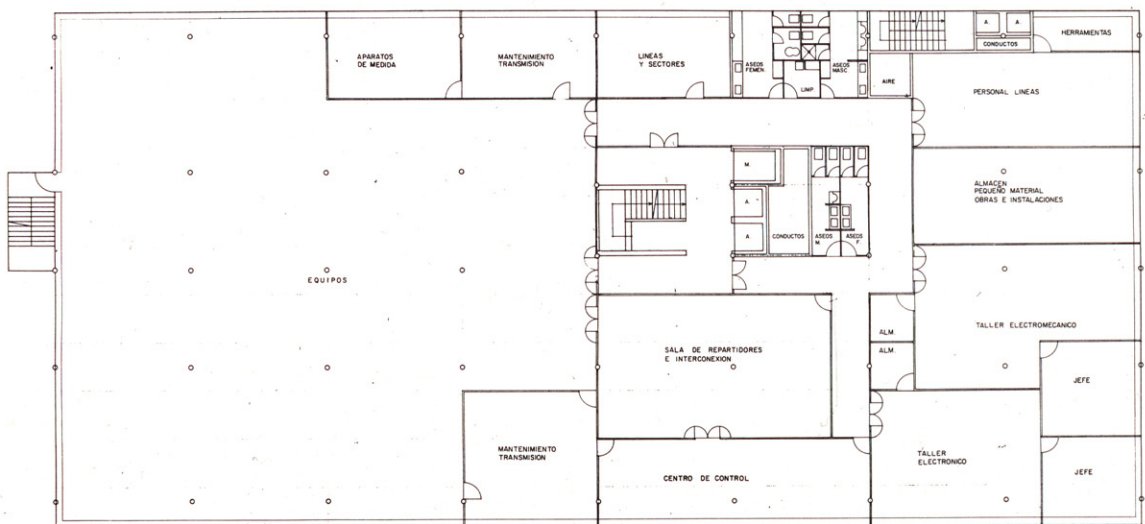
Planta segunda.
