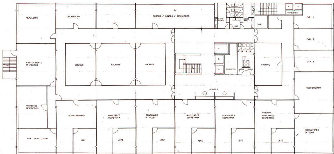
Planta segunda.
