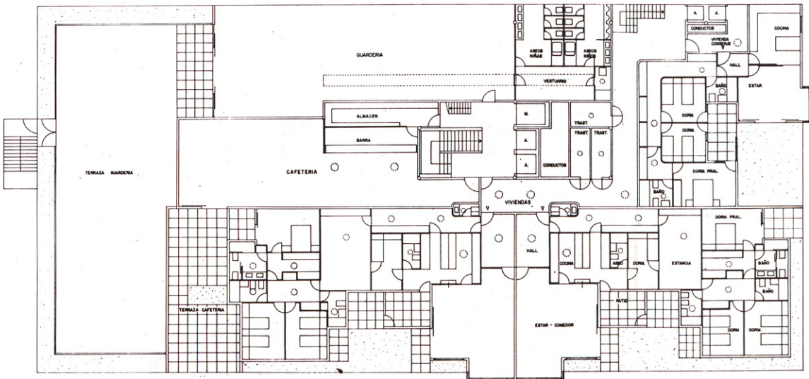
Planta cuarta.
