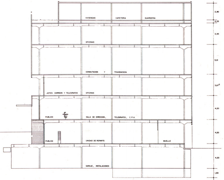
Sección.
