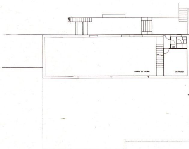
Planta sótano.
