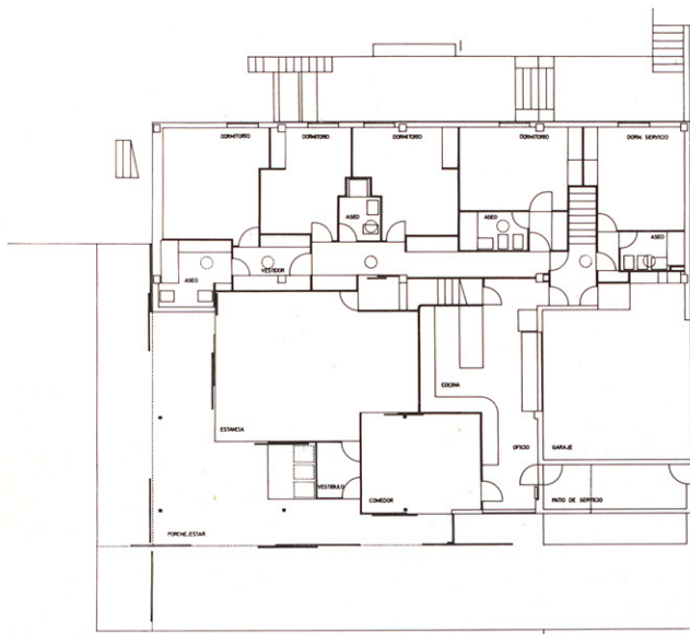
Planta baja.
