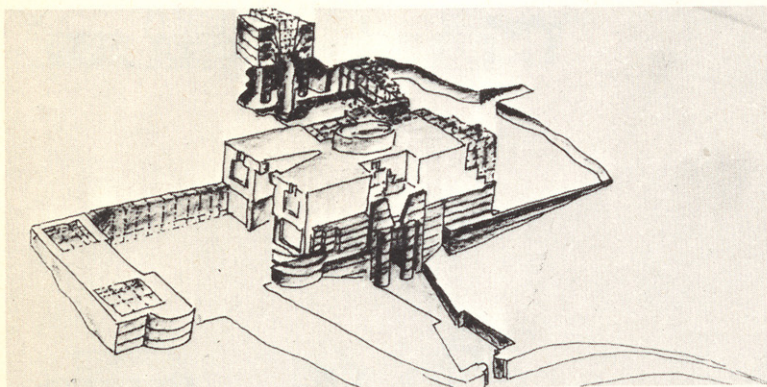
Plocek House, Princeton New Jersey, Michael Graves. Axonometría y estudio de la fachada.
