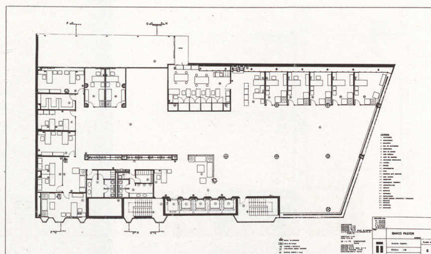
Planta cuarta
