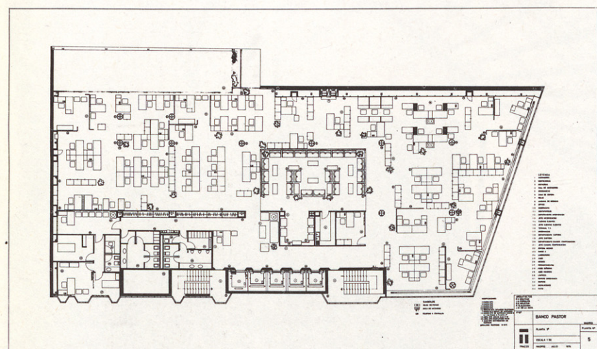
Planta tercera
