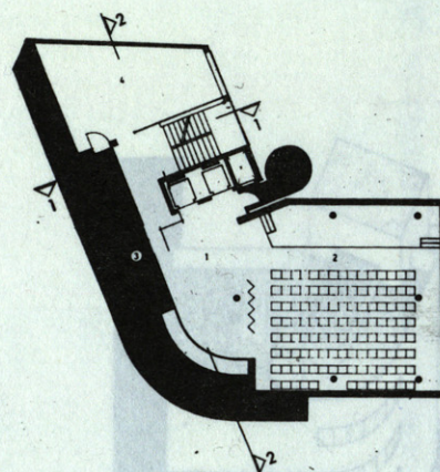
PLANTA 2 1 HALL 2 SALA DE ACTOS 3 ASIDOS 4 SALA DE REUNIONES
