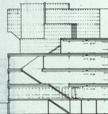
SECCIÓN BB
