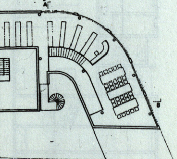
PLANTA 8 E 1:100 CEYS-BIBLIOTECA EQUIPO MECANICO
