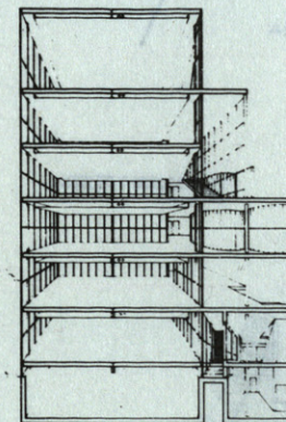
SECCIÓN AA
