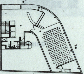
PLANTA 1 E 1:100 SALON DE ACTOS BAR
