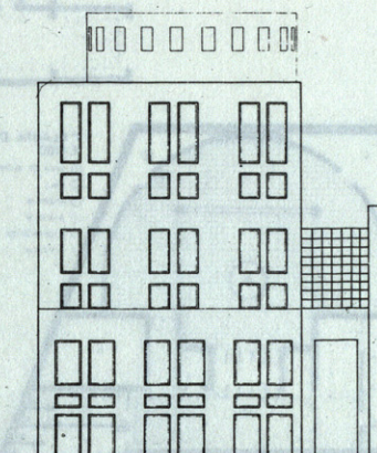
FACHADA A CALLE MERCEDES VELLIDA E 1100
