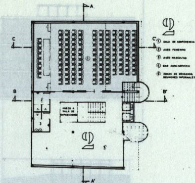
PLANTA 1ª
