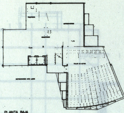
PLANTA BAJA
