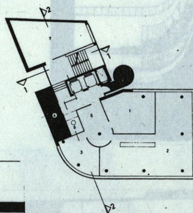
PLANTA 3 1 ASESORIA JURIDICA 2 DEPARTAMENTO SECRETARIA 3 HONORARIO 4 ASIDOS 5 ESPERA 6 CONFERENCIA 7 SALA DE REUNIONES
