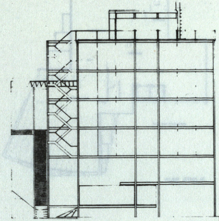
ALZADO PZA. SAN PEDRO
