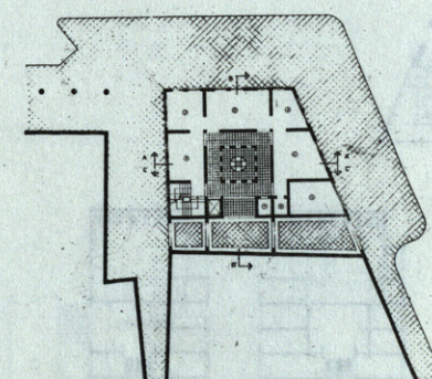
PLANTA BAJA E 1100
