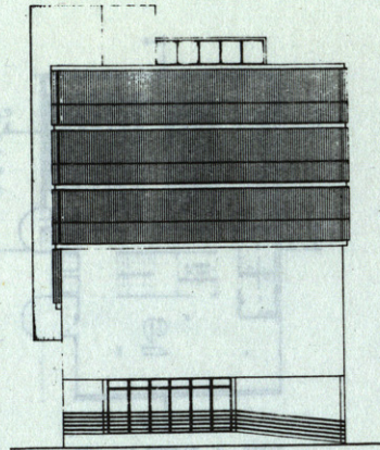
ALZADO PZA. SAN PEDRO
