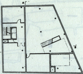
PLANTA -1 E 1:100 EXPOSICIONES ARCHIVOS ORDENADOR
