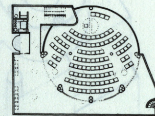
PLANTA 2 SALA DE REUNION SALA DE CONFERENCIAS
