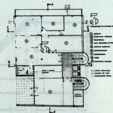
PLANTA 3ª
