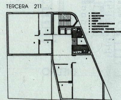
TERCERA 211
