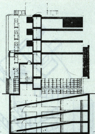
SECCION AB
