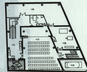
NIVEL -1
