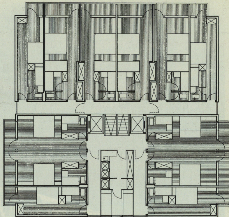
HOTEL MOUNTAIN AMINONA (Suiza) Planta tipo de un hotel con 180 camas en dos niveles.
