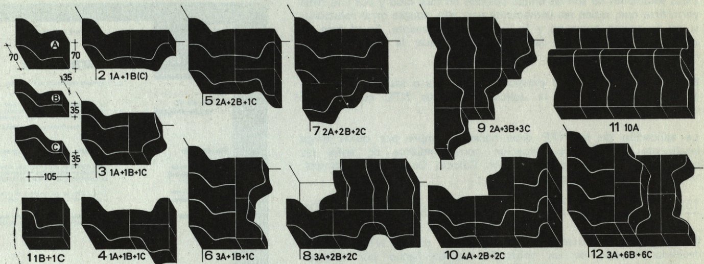
MATERIAL: ELEMENTOS DE ESPUMA DE POLIURETANO TAPIZADOS EN TEJIDO ACRILICO
