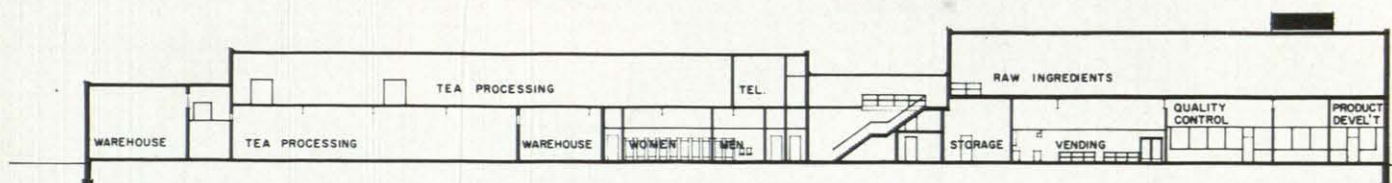
Sección.
