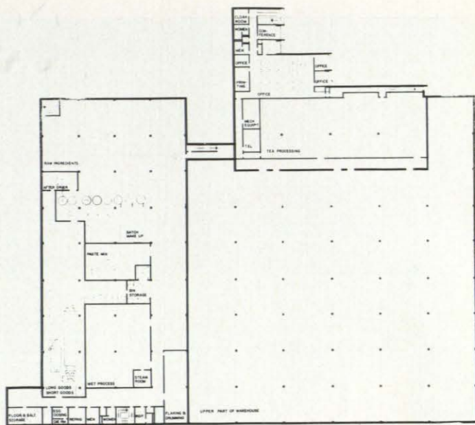
Planta segunda.
