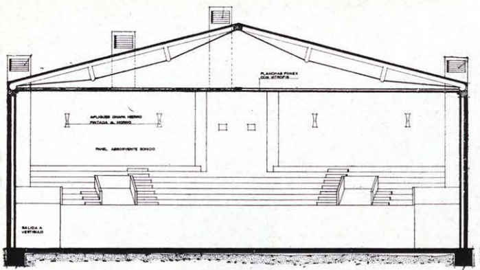
Secciones y planta del patio de butacas.
