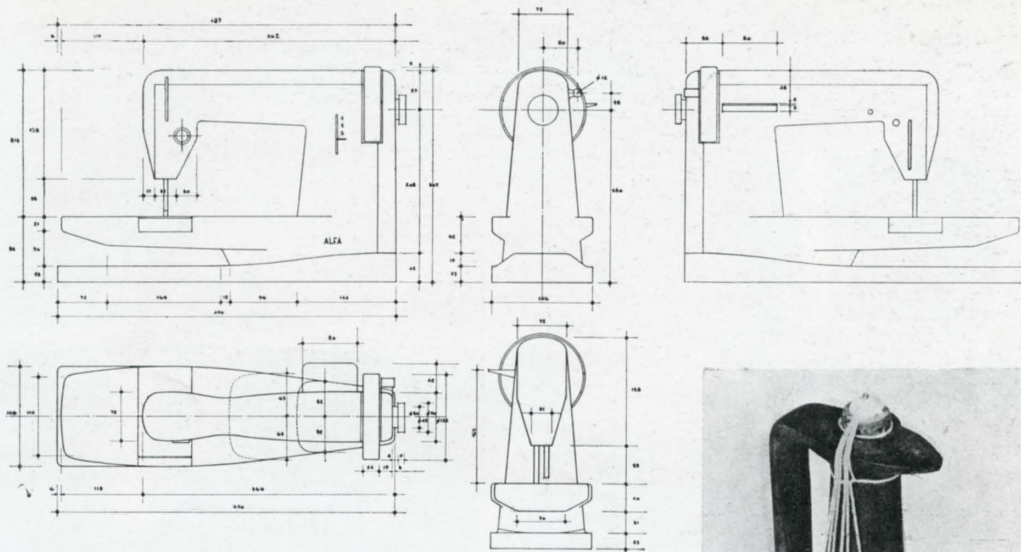
Planos de la máquina de coser Alfa y del motor para la misma. Proyecto: Javier Carvajal.
