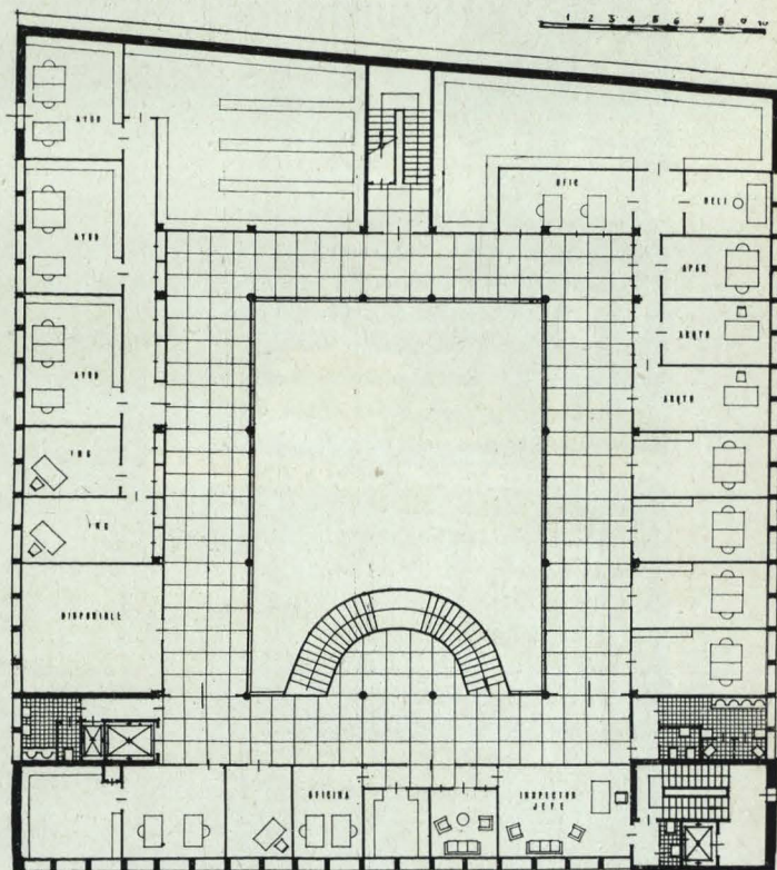
Planta tercera.
