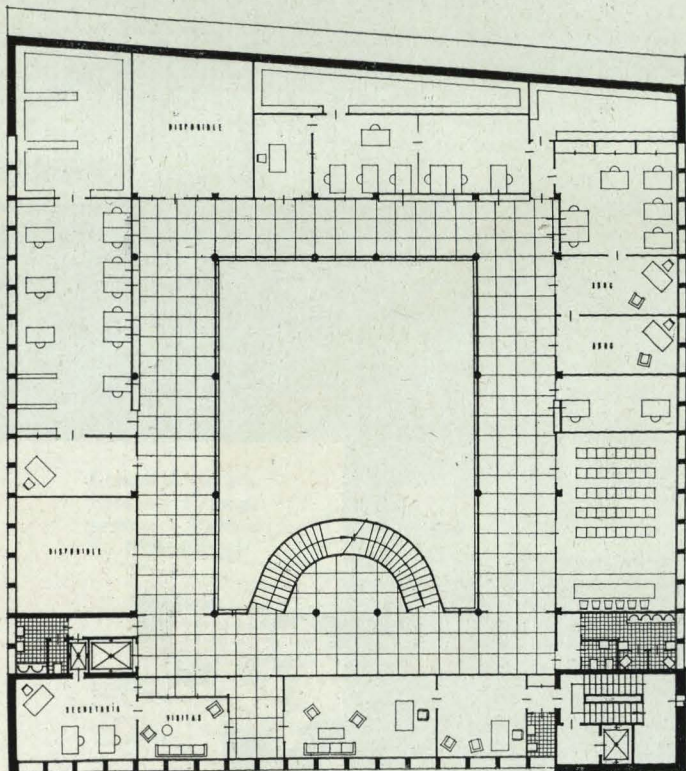
Planta segunda.
