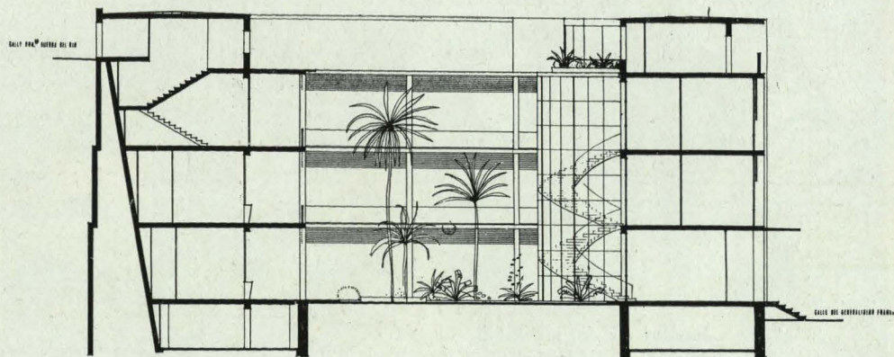
Sección transversal.
