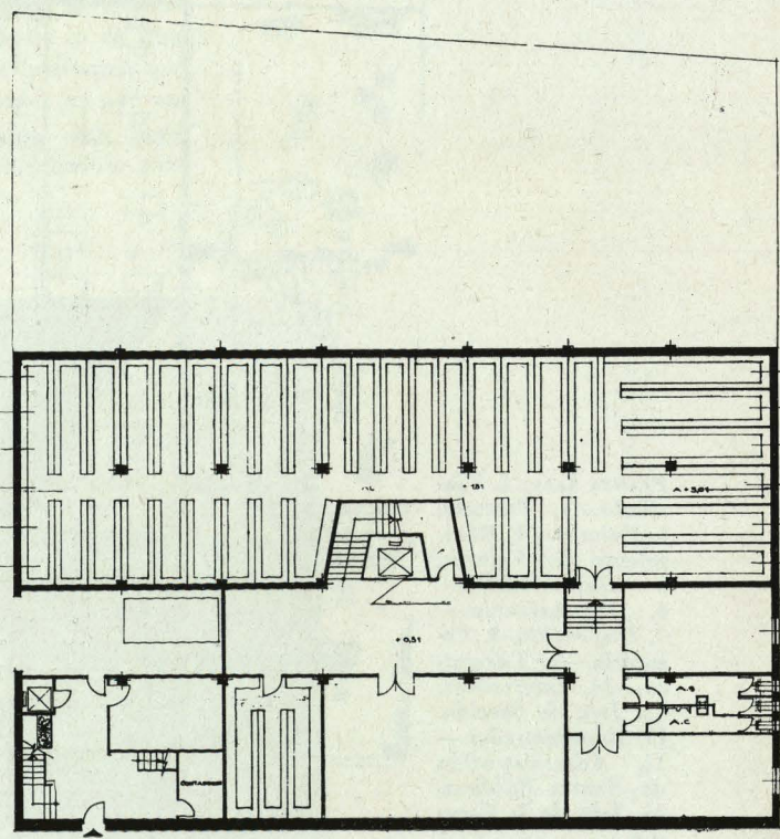
Planta sótano.
