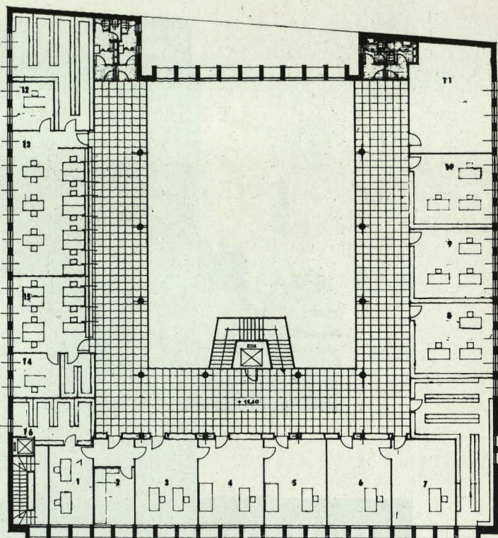
PLANTA SEGUNDA: 1. Dos Administrativos.—2. Delineante.—3. Aparejadores.—4. Arquitecto.—5. Arquitecto Jefe.—6. Ingeniero Jefe.—7. Ingeniero.—8. Conservación.—9. Conservación.—10. Conservación.—11. Disponible.—12. Administrador.—13. Administración de Propiedades y Contribución Territorial.—14. Jefe de Sección.—15.—16. Archivo.
