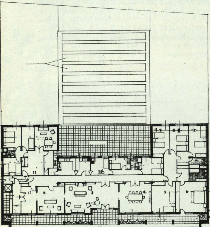
PLANTA TERCERA: 1. Hall.—2. Sala.—3. Estar.—4. Comedor.—5. Dormitorio.—6. Dormitorio.—7. Dormitorio.—8. Dormitorio.—9. Dormitorio.—10. Plancha.—11. Vestíbulo.
