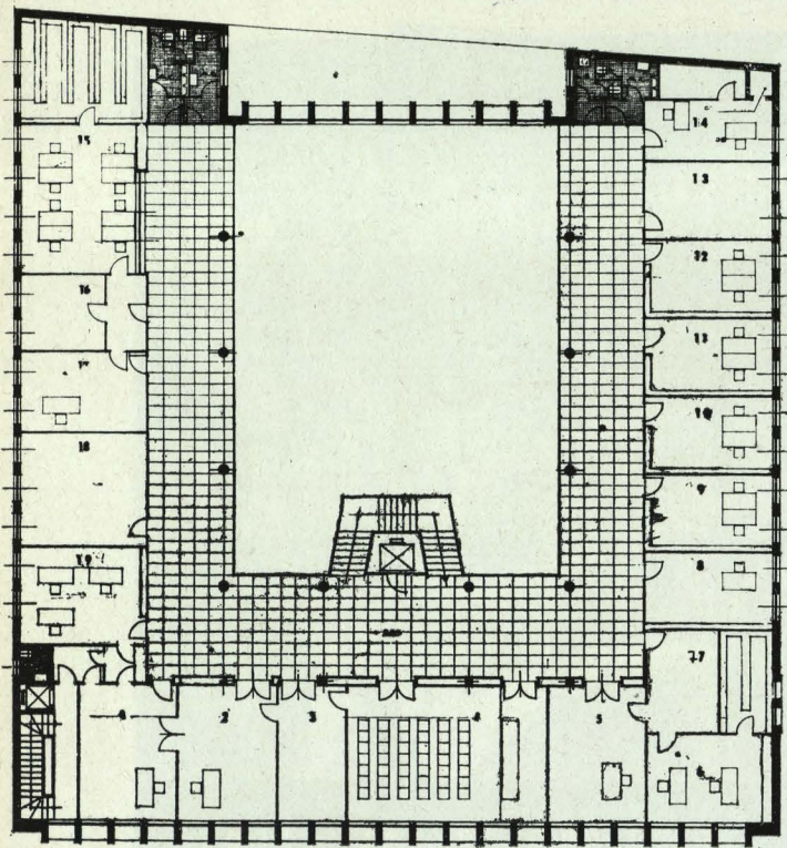
PLANTA PRIMERA: 1. Despacho de trabajo del Delegado.—2. Despacho oficial del Delegado.—3. Sala de visitas.—4. Salón de actos.—5. Inspector Jefe.—6. Dos funcionarios.—7. Visitas.—8. Inspector de Impuestos Especiales.—9. Dos Inspectores.—10. Dos Inspectores.—11. Dos Inspectores.—12. Dos Inspectores.—13. Disponible.—14. Dos funcionarios.—15. Abogacia del Estado.—16. Primer Abogado.—17. Abogado Jefe.—18. Disponible.—19. Secretario.
