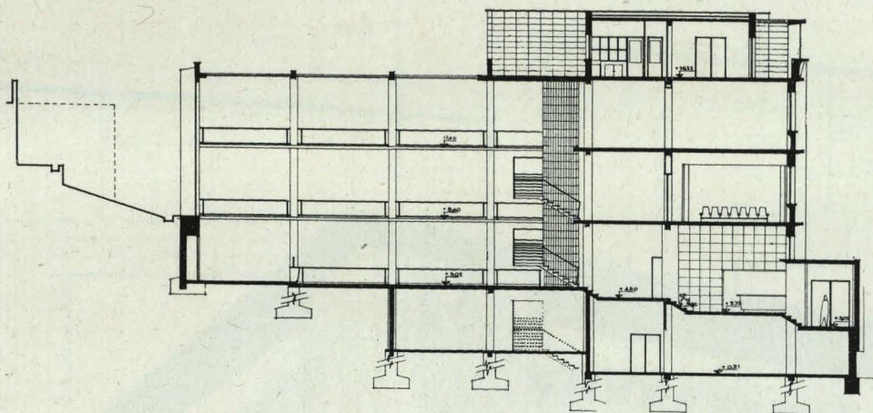
Sección.
