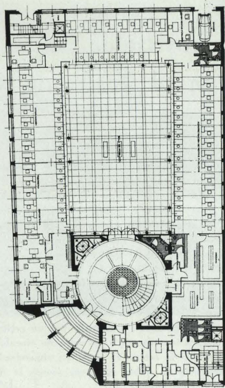
Planta primera.
