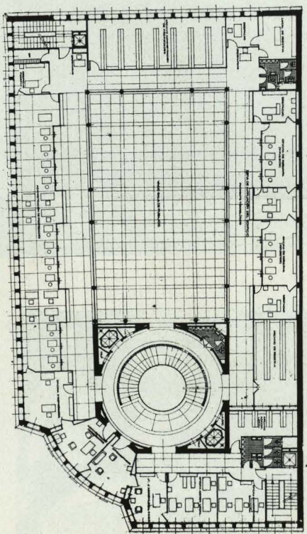
Planta segunda.
