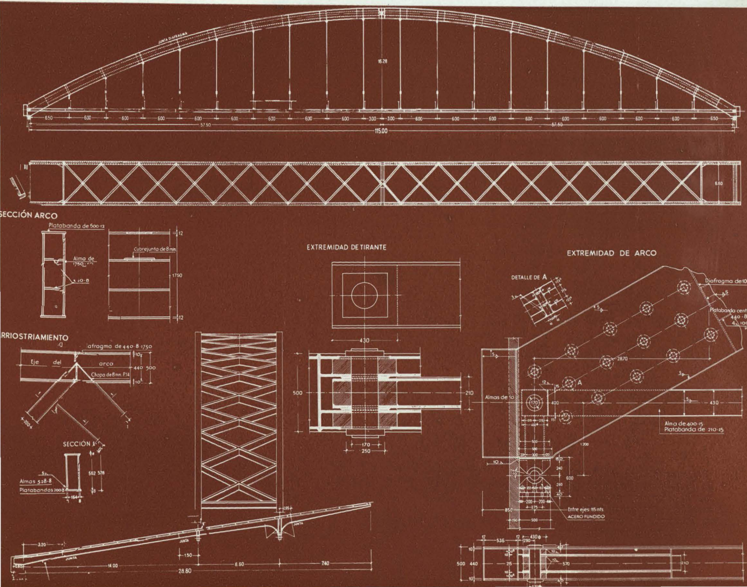
Vista de conjunto de la cubierta y detalles de las extremidades de arco y tirante.
