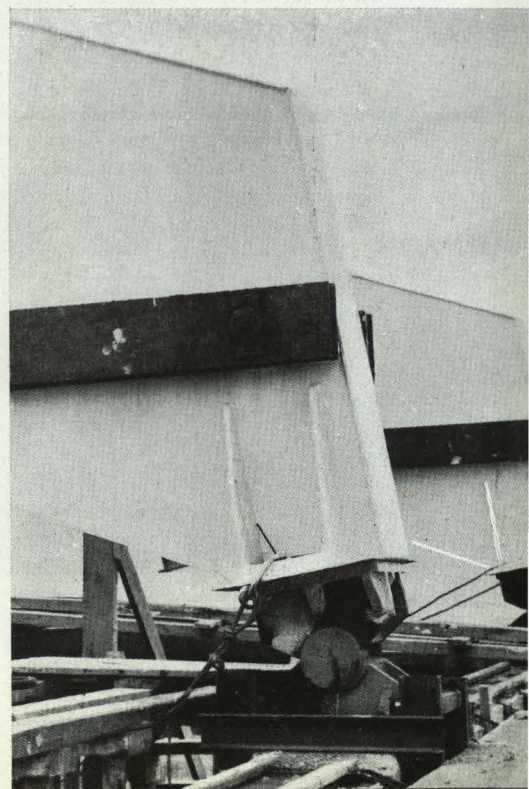
Las extremidades de los arcos con los carrones para su traslado.
