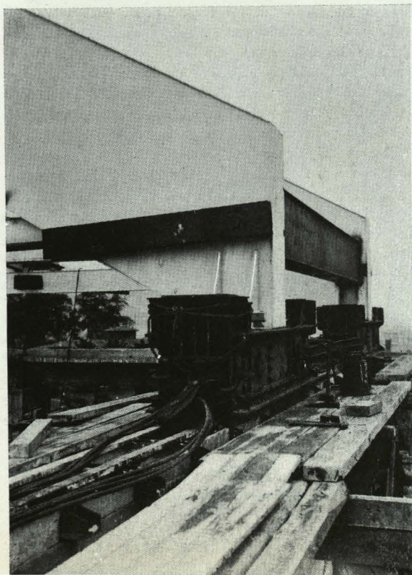
Las extremidades de los arcos con los carrones para su traslado.
