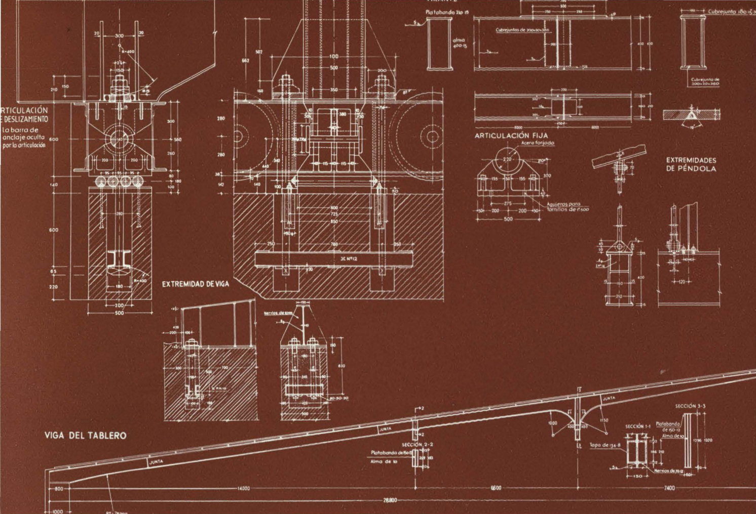
Detalles del tirante, péndolas, vigas del tablero y articulaciones de las extremidades de los arcos. (En la articulación móvil aparece el carrilón utilizado para el traslado de los arcos.)
