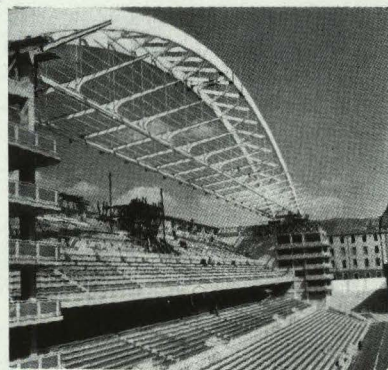
Vistas de la tribuna en diferentes fases de la obra desde la tribuna llamada de "gol".
