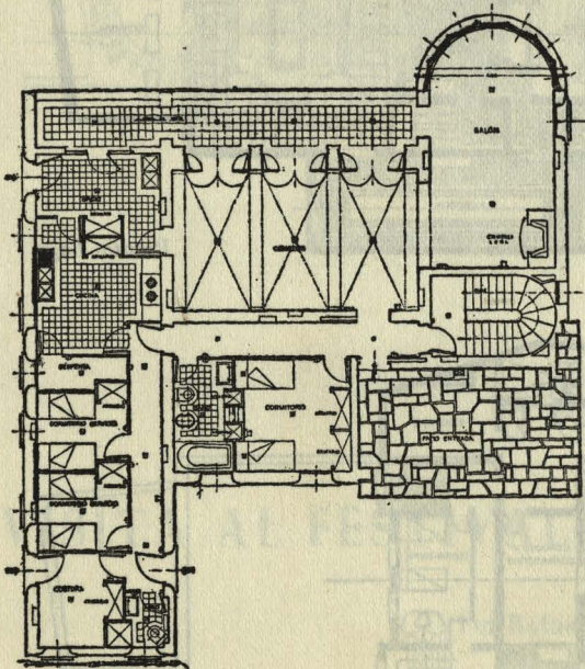
Planta baja.
