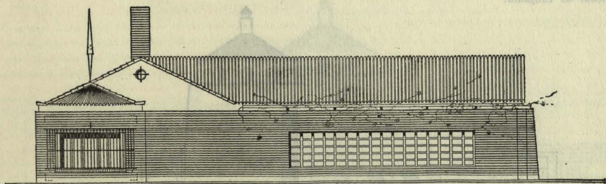
Fachada Oeste.
