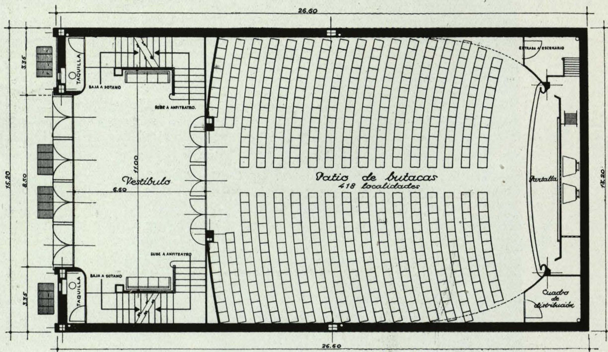
Planta del patio de butacas
