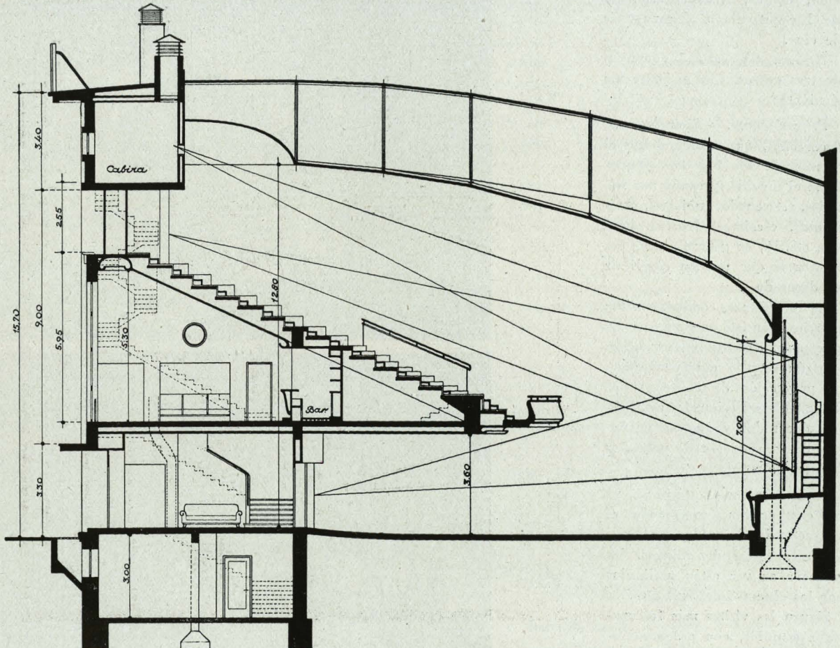
Sección longitudinal
