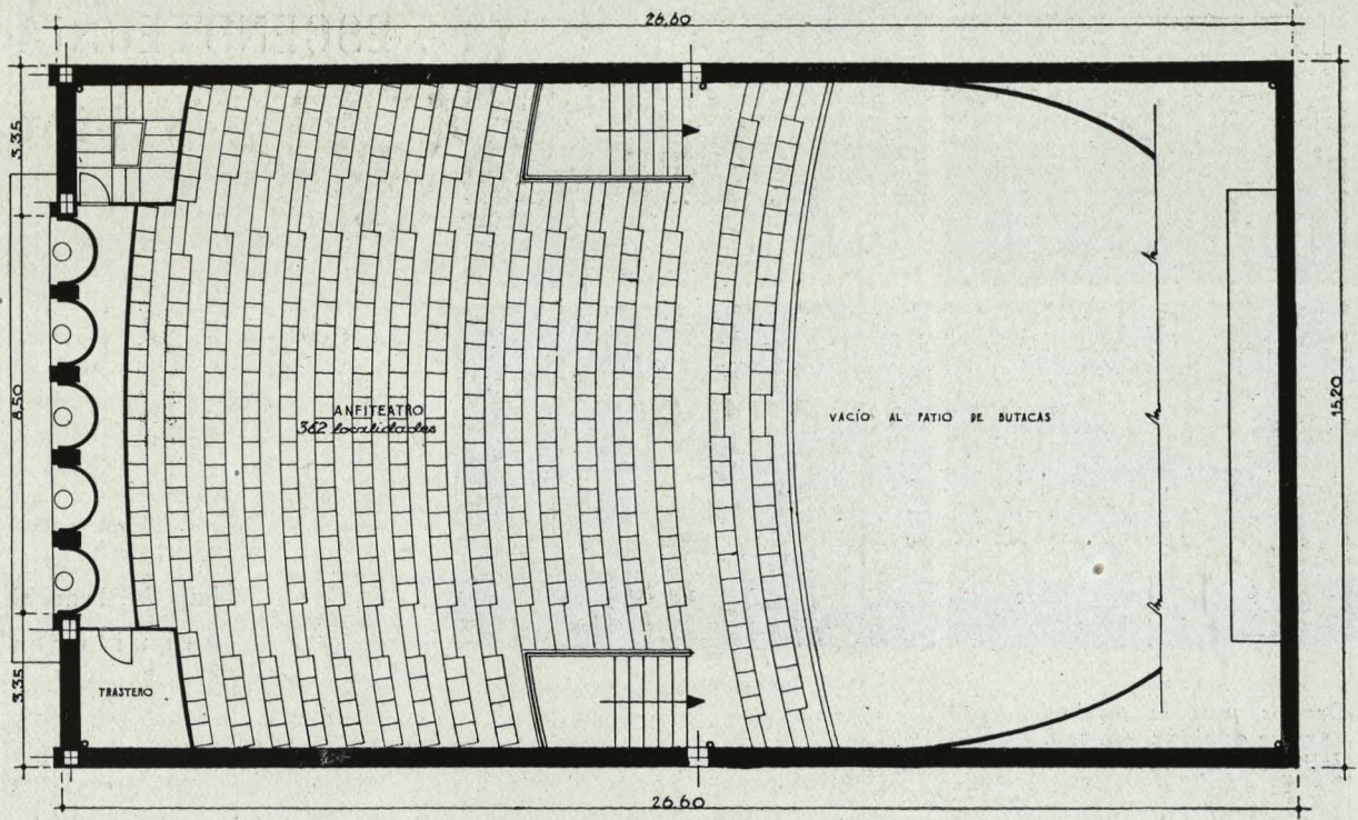
Planta de anfiteatro
