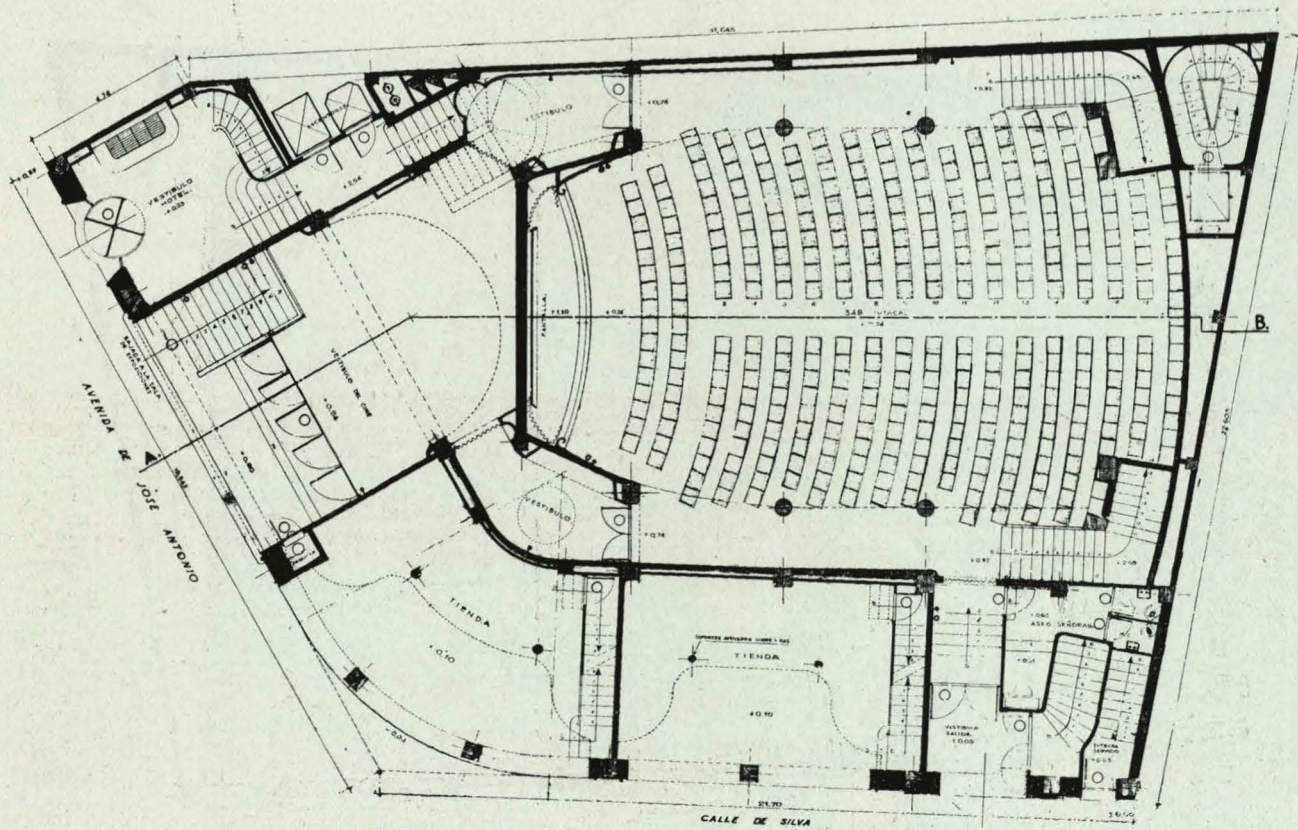
Planta del patio de butacas.
