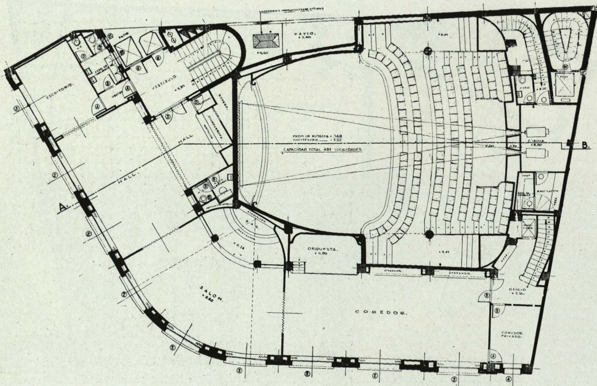
Planta de anfiteatro.
