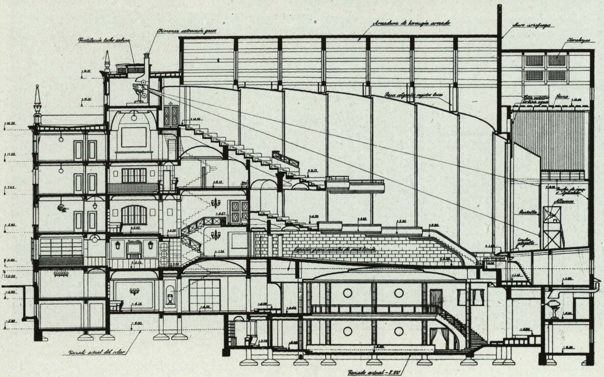
Sección longitudinal.
