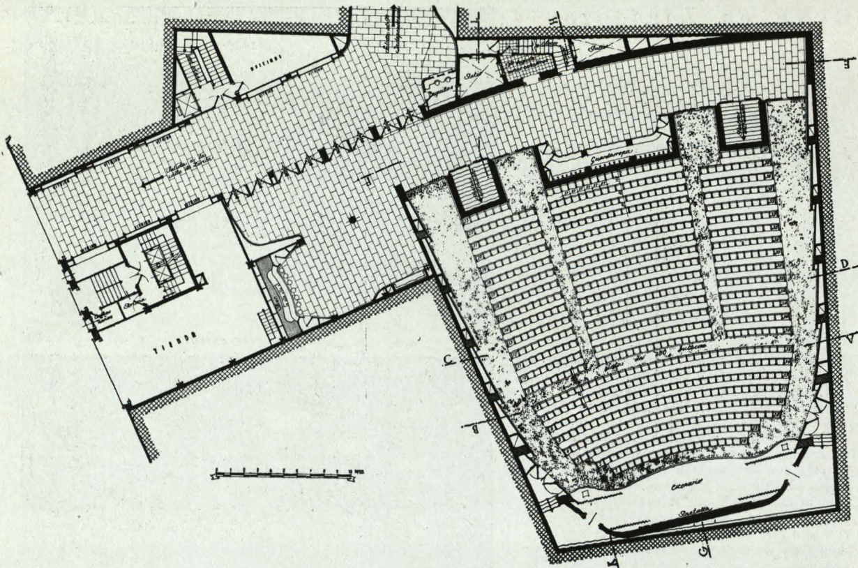
Planta baja y secciones.
