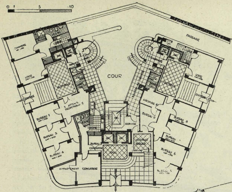
Planta baja.
