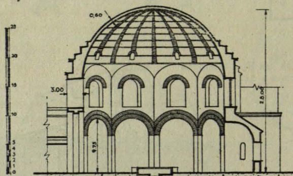
TEMPLO DE LA MINERVA MEDICA AÑO 263 a 268.
