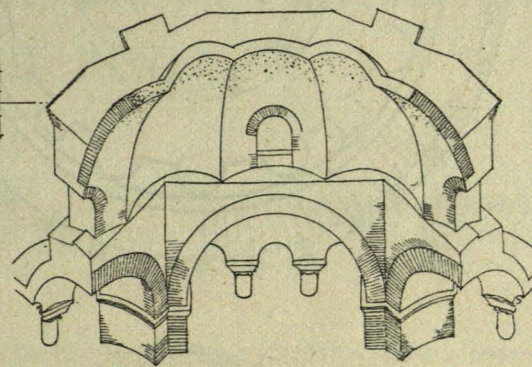
TEMPLO DE SAN VITAL DE RAVENA AÑO 526 a 547 .
