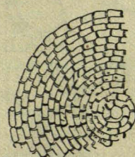
DETALLES DE LA CÚPULA DE ALFARERIA .
