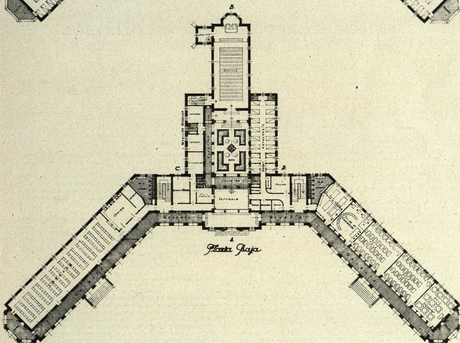
Plantas del Orfelinato "Legionarios de Franco".
