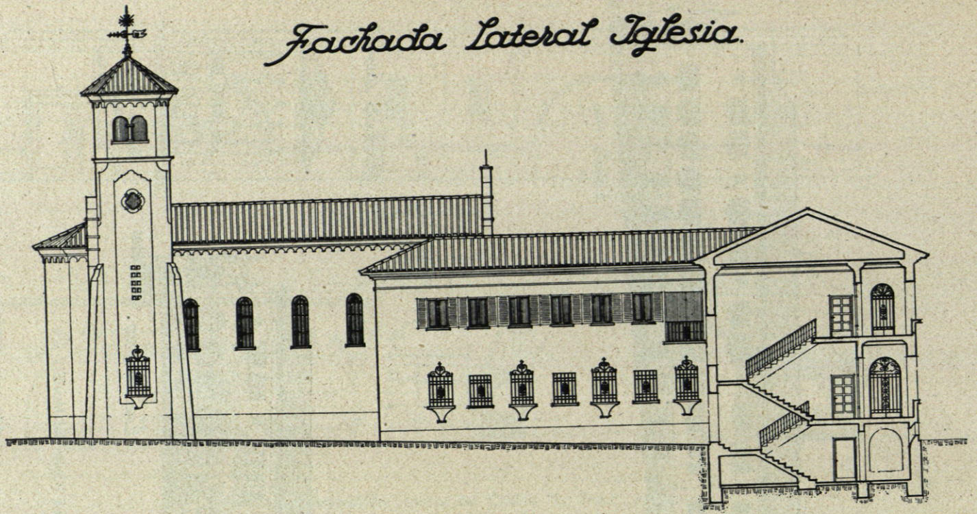
Proyecto del Orfelinato "Legionarios de Franco".
