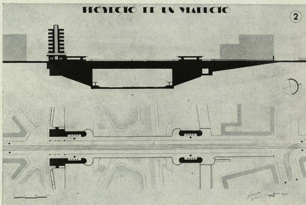
Proyecto de un Viaducto. Martín Aguirre, arquitecto; R. M. Ceballos, Ing. de Caminos.
