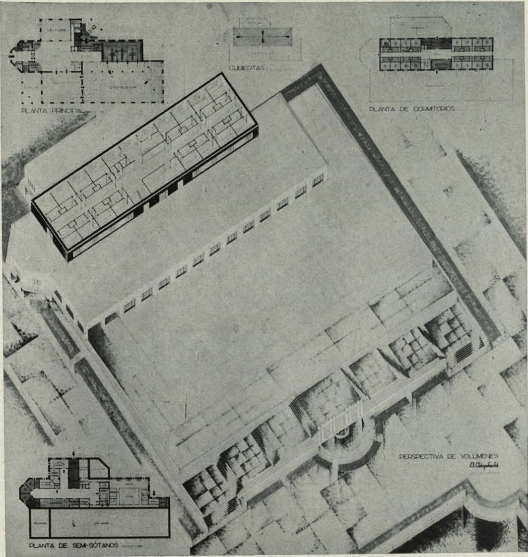
Luis G. de la Rasilla: Estudio para el proyecto de un Restaurant con Hotel de viajeros en Aranjuez.
