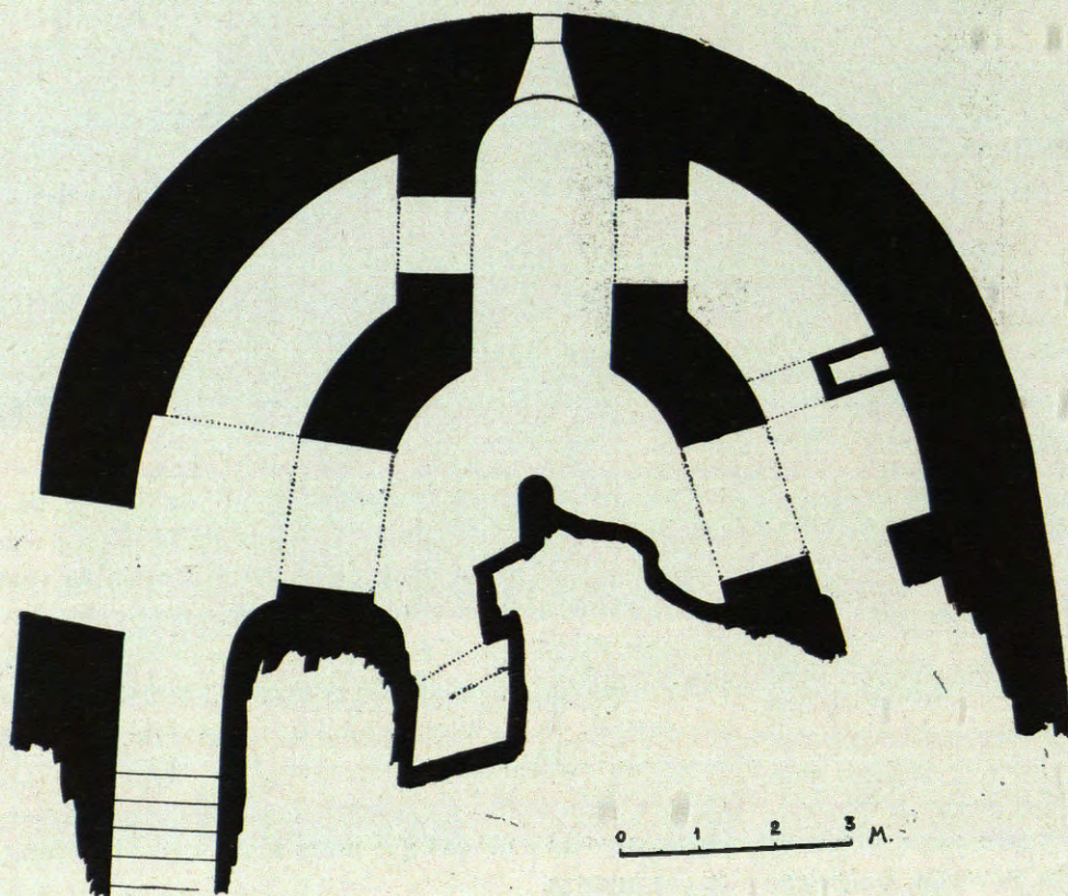
PLANTA DE LA CRIPTA DE LA IGLESIA DE SAN PEDRO DE RODA (GERONA)
