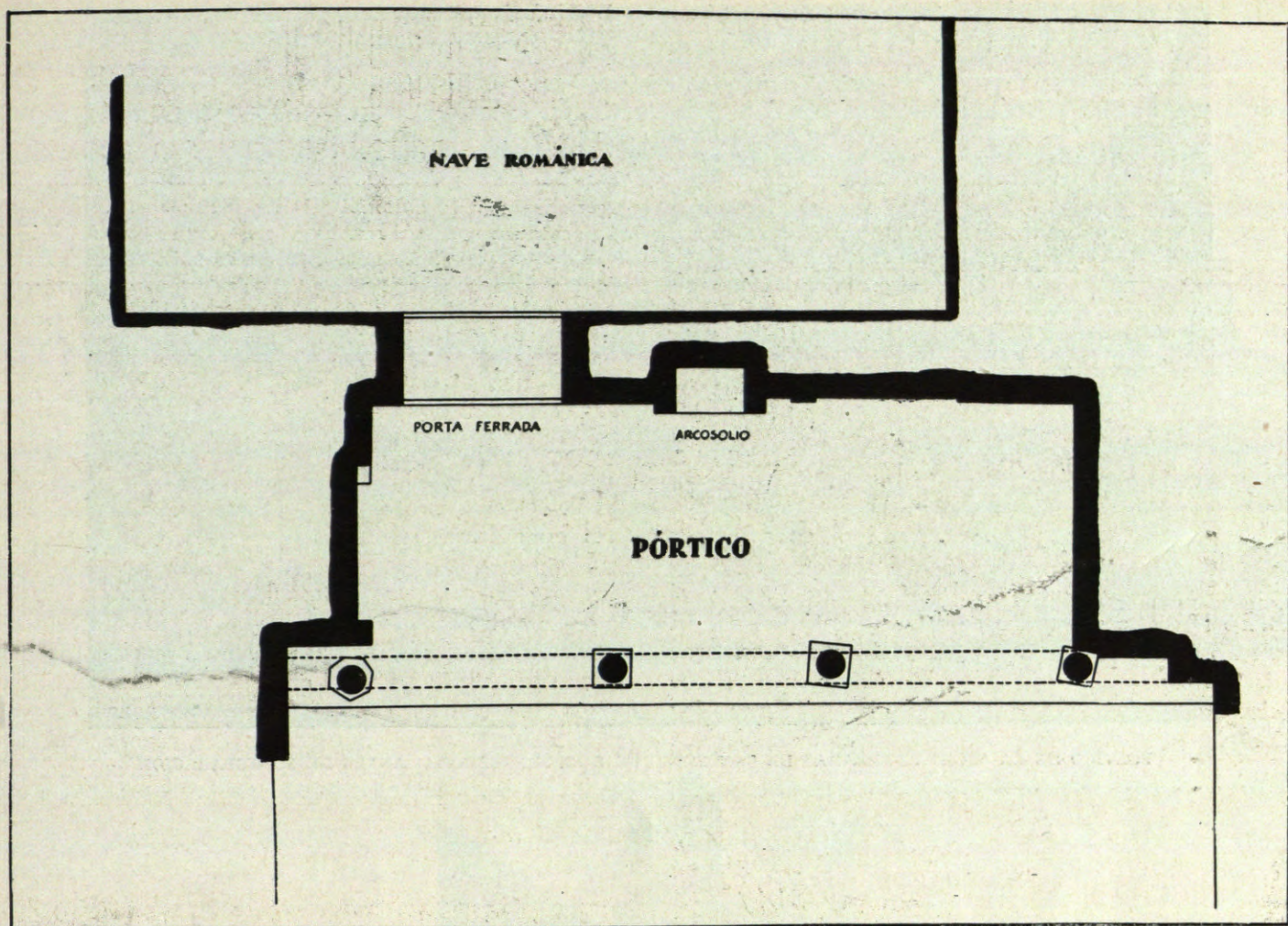
PLANTA DEL PÓRTICO DE SAN FELIU DE GUIXOLS (GERONA)
