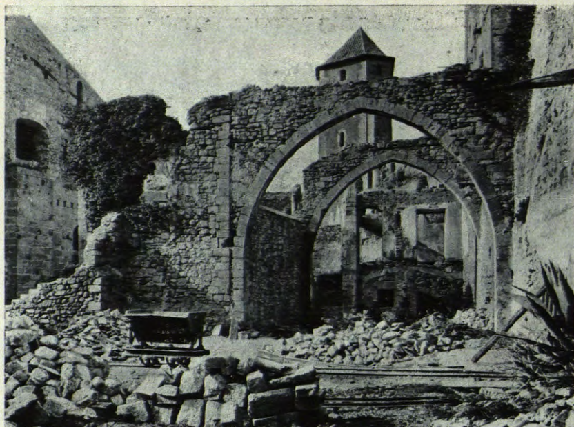
MONASTERIO DE POBLET (TARRAGONA). ARCOS ADOSADOS A LA MURALLA DE PEDRO III, LOS CUALES ESTABAN TAPIADOS Y HAN SIDO DESCUBIERTOS, DESPUES DE SU CONSOLIDACION
