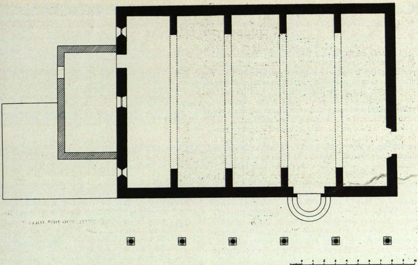
PLANTA DE LA IGLESIA DE SAN FELIX (JATIVA)
