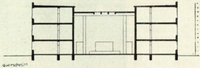
querschnitt
