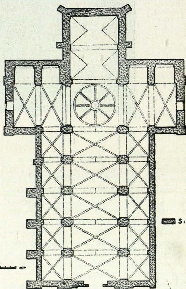
PLANTA DE LA IGLESIA DE MONTEDERRAMO
