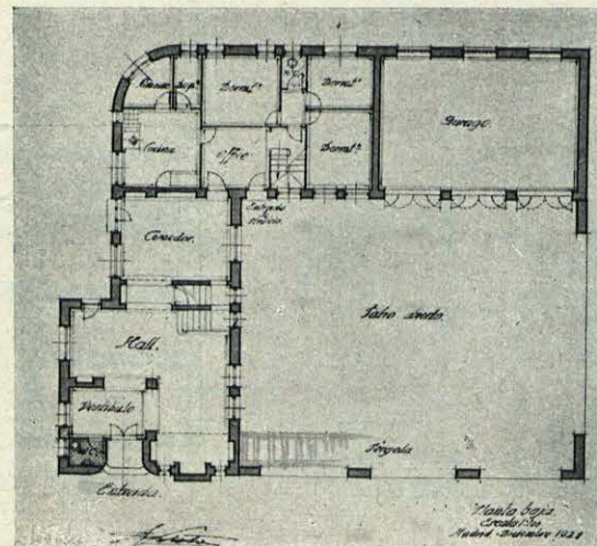
PROYECTOS DE LOS SRES. FEDUCHI, VILATA Y ECED. DOS SOLUCIONES (SEGUNDO PREMIO).
