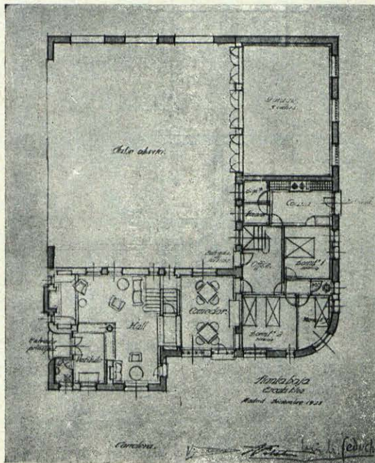
PROYECTOS DE LOS SRES. FEDUCHI, VILATA Y ECED. DOS SOLUCIONES (SEGUNDO PREMIO).
