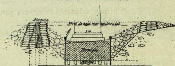
Sección transversal
