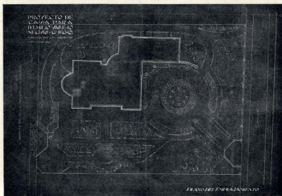
CASA PARTICULAR EN NEGURI (BILBAO).—INGRESO POSTERIOR Y PLANTA DE EMPLAZAMIENTO.
