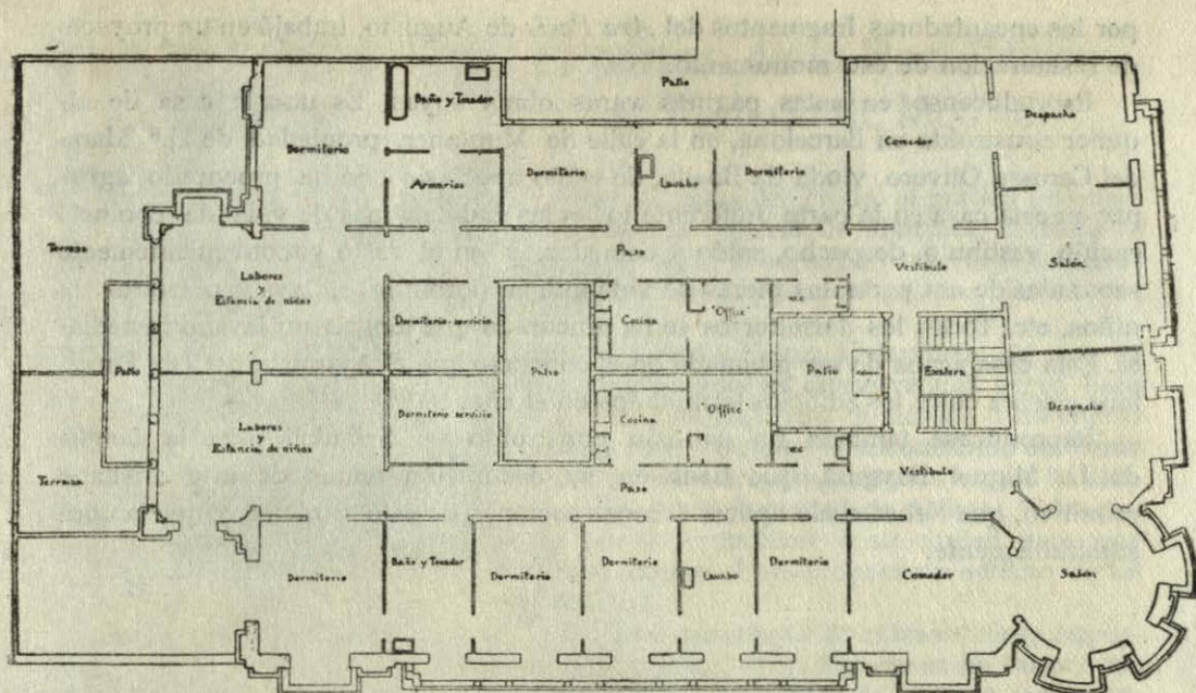
Casa en la calle de Muntaner, Barcelona.—Planta del piso principal.—Arquitecto: F. de P. Nebot.
